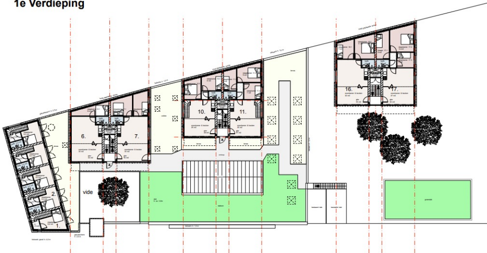
1e Verdieping
